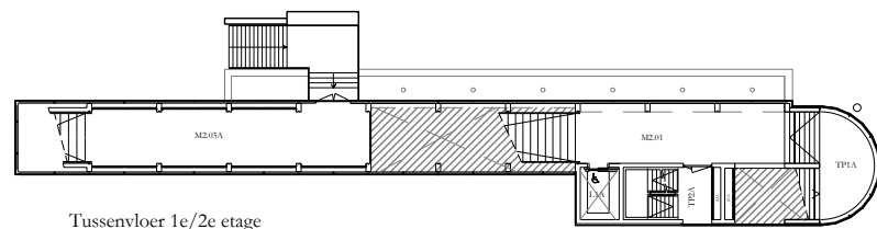
Tussenvloer 1e/2e etage
