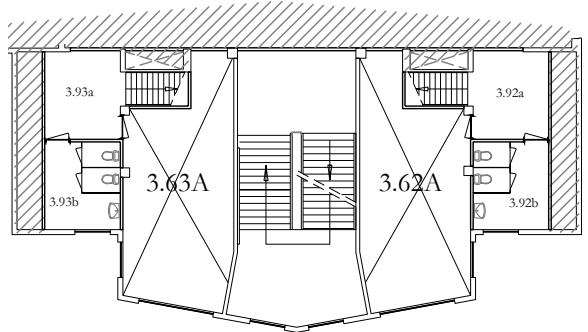
Tussenvloer 2e - 3e etage
