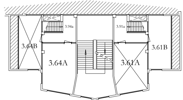
Tussenvloer 3e - 4e etage
